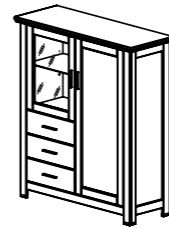
Typ 45 B/H/T 1327/1496/480
