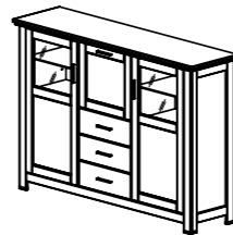
Typ 47 B/H/T 1866/1298/480
