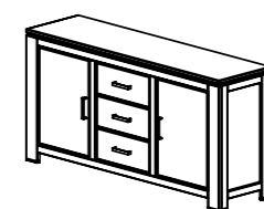
Typ 48 B/H/T 1748/871/470
