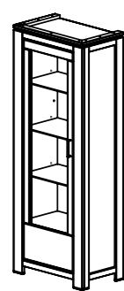
Typ 10 B/H/T 780/2055/470
