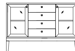
komoda przeszklona [P-24] szer. 157/gł. 46/wys. 108 cm
