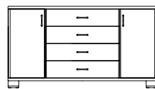
komoda duża Edel [E-7] szer. 141/gł. 43/wys. 77 cm
