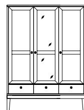
szafa 3D [P-19] szer. 148/gł. 60/wys. 200 cm
